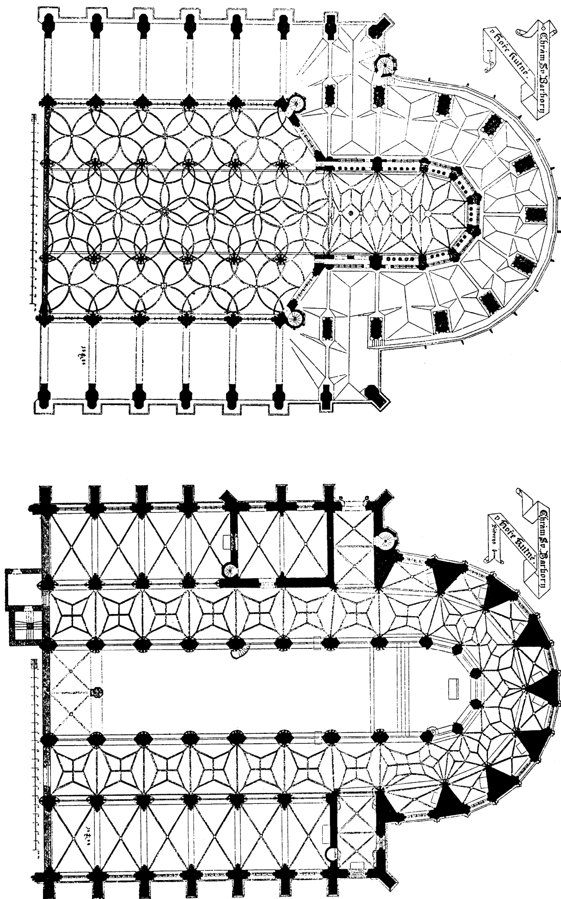
Půdorys chrámu sv Barbory v Kutné Hoře z roku 1886 (Dole půdorys přízemí, nahoře půdorys ve výši chóru)
