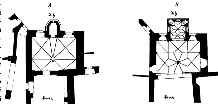
Obr. 1. Půdorys. (A přízemí, B patro)
