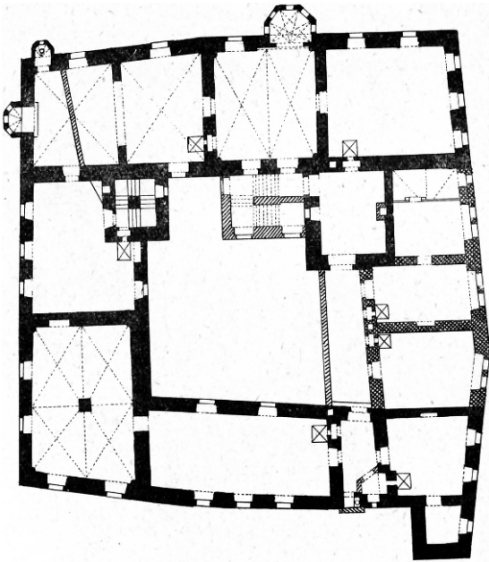
Půdorys Hrádku v poschodí z r. 1837.
