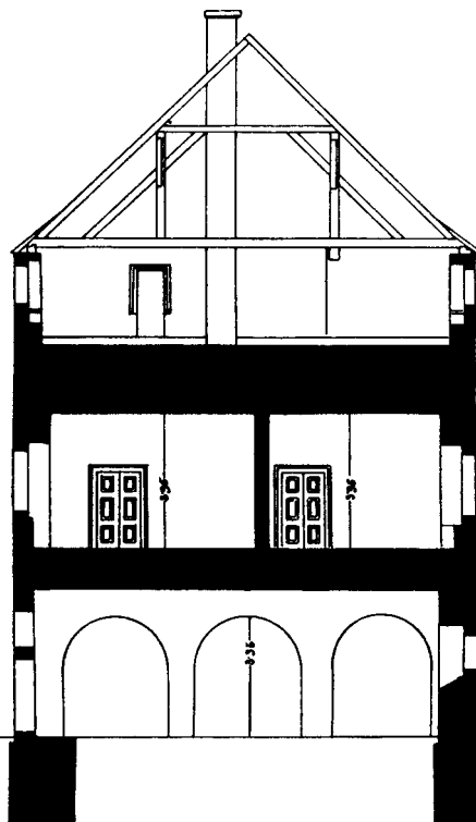
Obr. 33. Řez vysokým domem.
