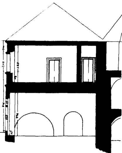
Obr. 19. Řez šmitnou a býv. kanceláří mincmistrovou.
