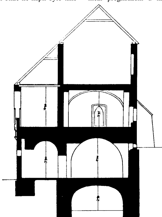
Obr. 31. Řez komorou, rejtunkem a puchalterií.
