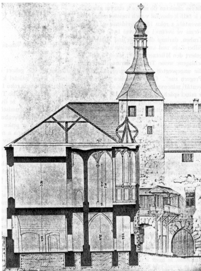
Obr. 24. Řez mincí a kaplí.
